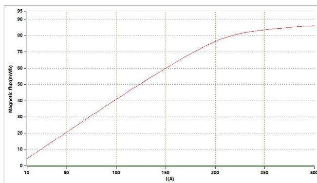
磁链图
