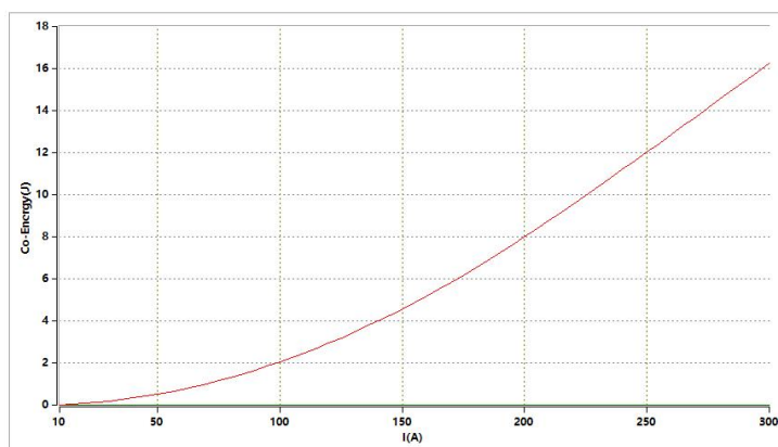
磁共能图
